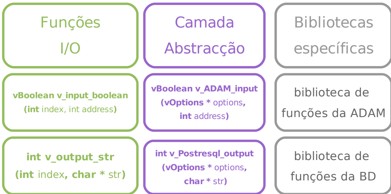
Figura 3.5 – Modelo de funcionamento da camada de comunicações
